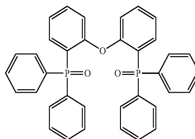
DPEPO
