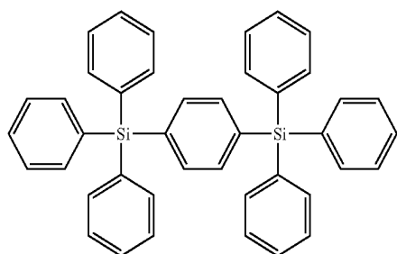
UGH2
