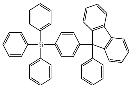
TPSi-F
