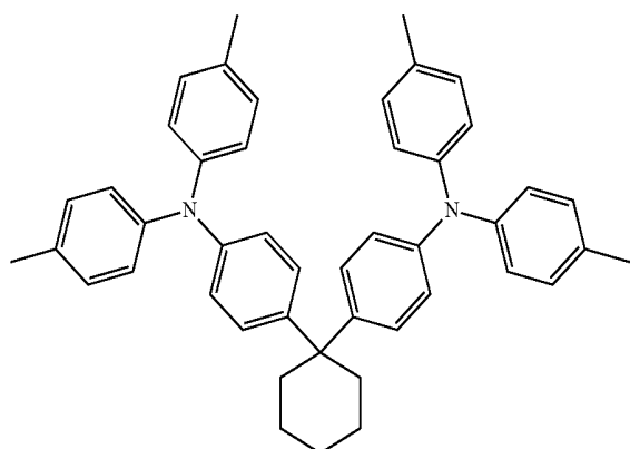
TAPC
